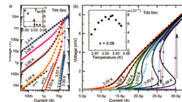
图二: TiN 薄膜在不同温度下的 I-V 曲线。(a) 在双对数标度下的 I-V 曲线。点虚线对应 V \propto I^\alpha , \alpha = 3 , 虚线对应 \alpha = 1 。插图显示 \alpha 指数对温度的依赖关系,箭头标记的温度是 BKT 相变温度,对应 \alpha = 3 , TBKT = 3.03 K。(b) 线性标度下的 I-V 曲线。实线是理论曲线。箭头标记电压的跳跃: 电流从零增加时候,对应的是电压向上的跳跃; 电流减少时候,电压会向下跳跃。
