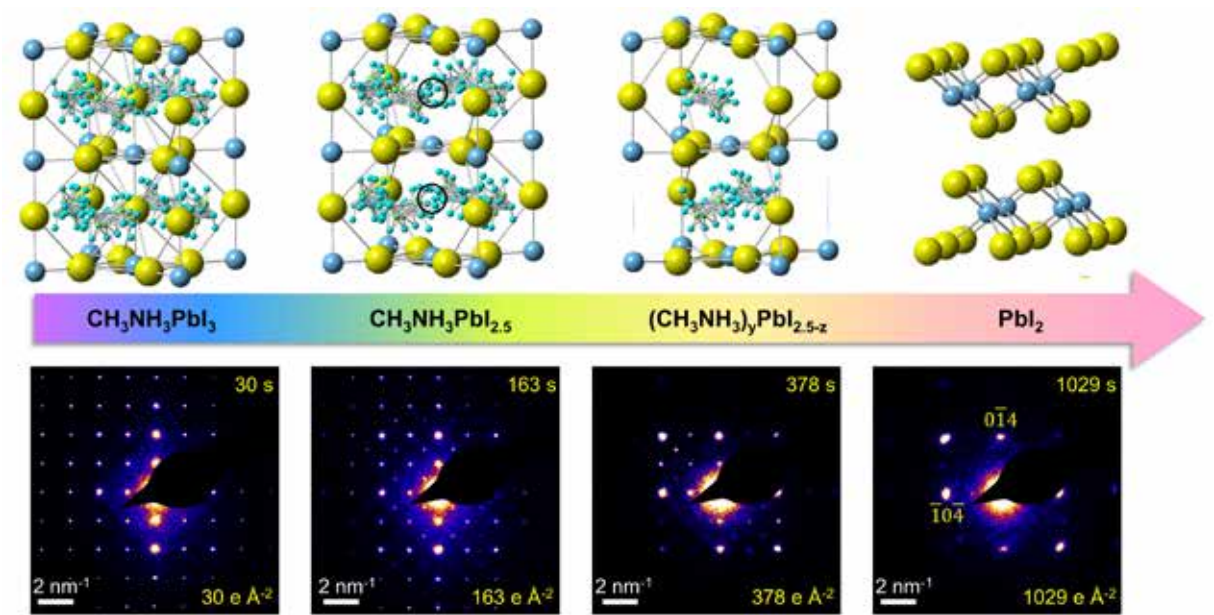
图：钙钛矿在电子束辐照下的分解路径。 Fig. The decomposition pathway of MAPbI 3 under electron beam illumination.
