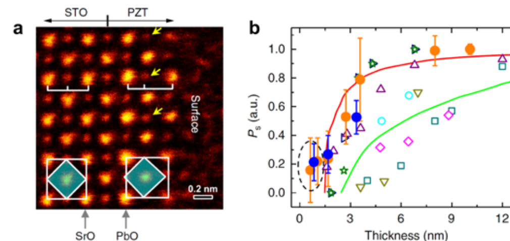
图二 . (a) 环形明场像的 1.5\text{ u.c.} ( 0.6\text{ nm} ) \text{PbZr}_{0.2}\text{Ti}_{0.8}\text{O}_3 (PZT)/STO 薄膜，使用了伪色以清晰展示各原子。（b）不同薄膜厚度下极化大小的比较，其中蓝色和橙色实心圆点数据来自本工作。
