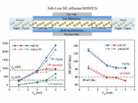
图 2. 单层碲烯晶体管示意图与性能
