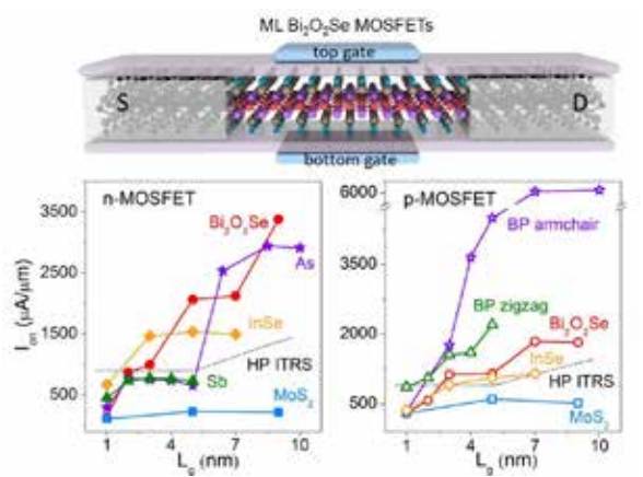
图 1. 单层 Bi 2 O 2 Se 晶体管示意图与二维晶体管性能比较。
