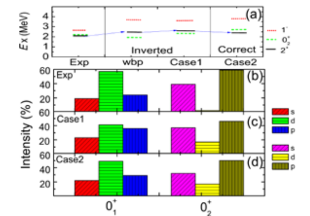
图 2: (a) 对于 ^{12}\text{Be} 低占据态，实验测量和壳模型计算（wbp 或者 YSOX 相互作用）的能级对比图。(b) 对于 ^{12}\text{Be} 的 0^+_{1,2} 态，实验测量的 s-, p-, d- 波强度。(c) 利用壳模型和 YSOX 相互作用，计算得到的 s-, p-, d- 波强度 (case1)。(d) 同图 (c)，但是 YSOX 相互作用中，d- 轨道降低了 0.5 MeV (case2)。
