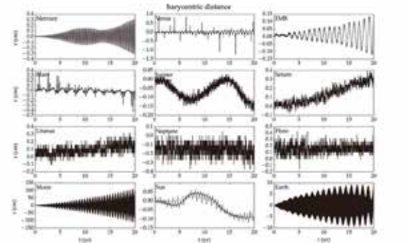
图二、李柯伽团组的太阳系动力学模型和 JPL DE435 的行星位置比较（Guo et al., 2019, MNRAS）。
