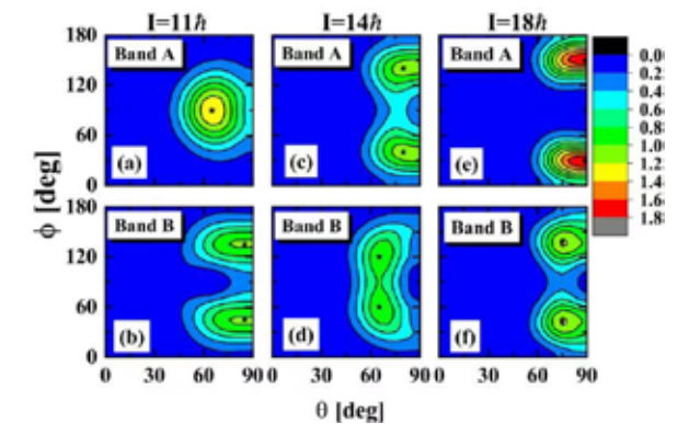
图 2. A-Plot，即原子核角动量在 ( \theta, \phi ) 平面上的取向分布。图中展示对于原子核 ^{128}\text{Cs} 中的手征双重带（带 A 和带 B），角动量投影方法给出的自旋 I 为 11\hbar [(a), (b)], 14\hbar [(c), (d)], 和 18\hbar [(e), (f)] 时的角动量取向分布。
