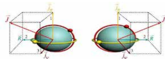
图 1. 原子核中的左手和右手手征几何。
