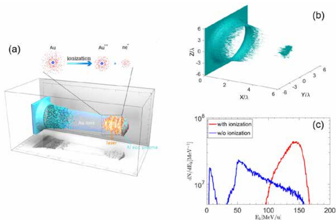
图1 (a) 光压加速动态致稳方案示意图；(b)和(c)分别展示三维粒子模拟结果：(b)带有Au涂层的Al靶加速后Al 13+ 离子密度分布，(c)考虑(红线)和不考虑(蓝线)动态电离，最终获得Al 13+ 离子能谱。
