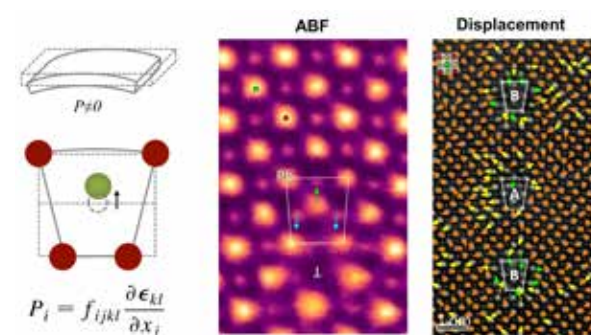
图一 . 由于挠曲电效应，应力梯度导致的结构畸变从而产生电极化。（左）原子尺度的挠曲电效应示意图。 \text{SrTiO}_3 中位错核附近的（中）结构畸变和（右）原子位置偏移。
