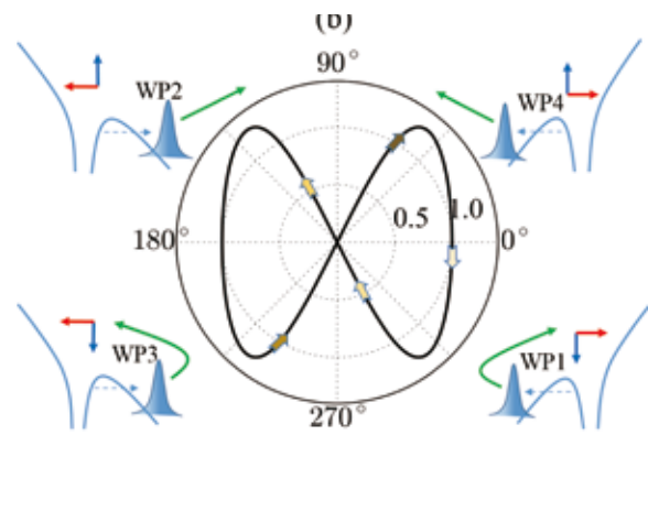
图 1 等强度偏振正交的 800nm 和 400nm 激光的合成光场的时空结构以及在激光场最大值处的量子隧穿示意图
