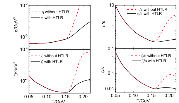
图 2. 剪切粘滞系数 \eta 和体粘滞系数 \zeta 及它们与熵密度的比值随温度的变化行为的计算结果。
